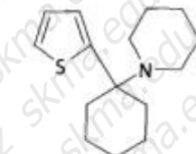
тиеноциклин 1-(2-тиенил)-цикло- гексил-пиперидин
